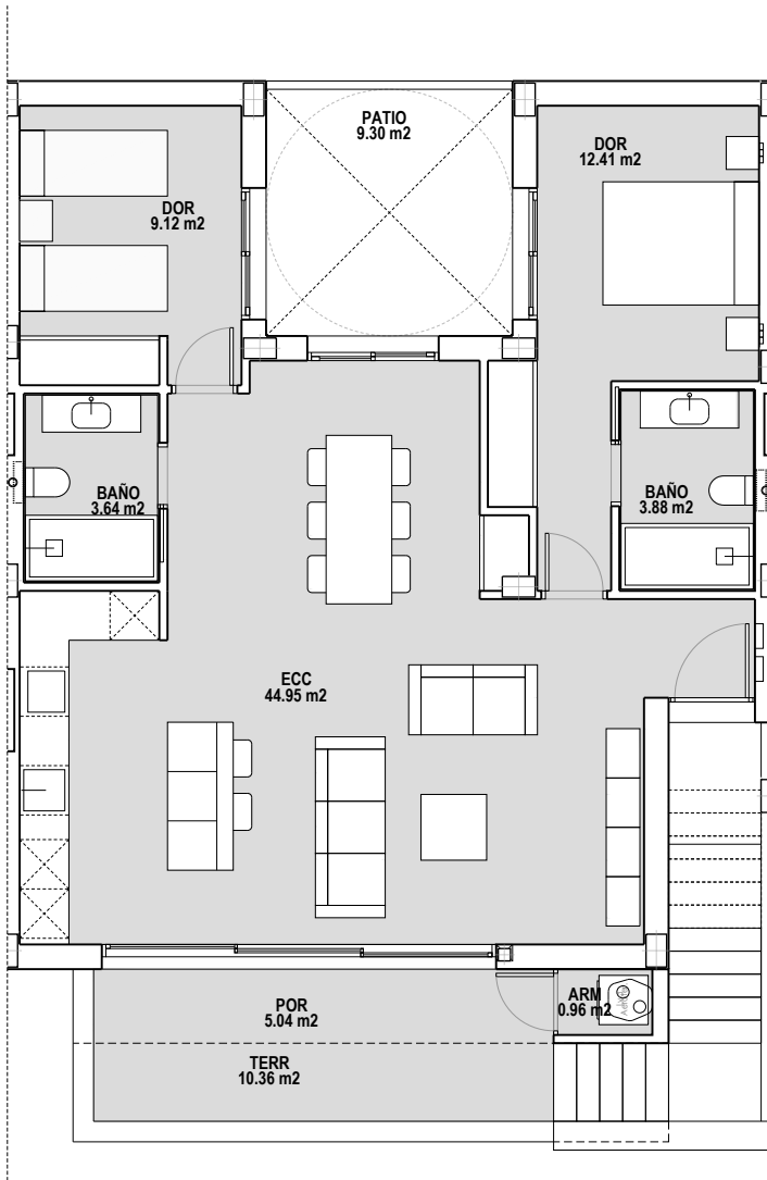
Vivienda 9/ alternativa
